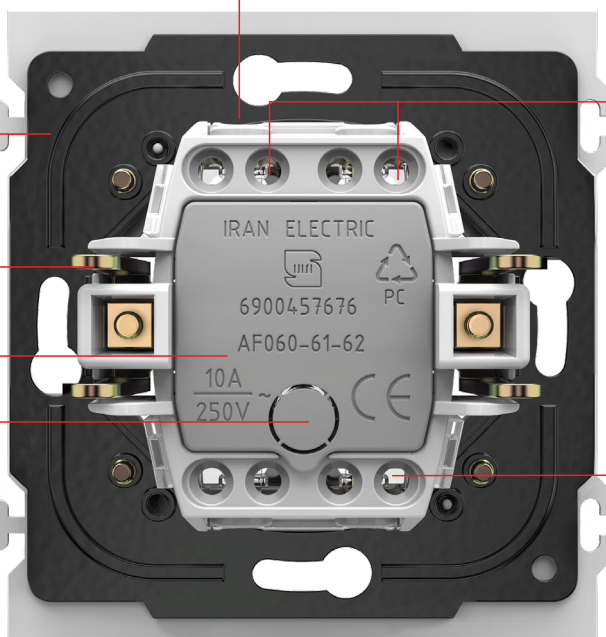
پیچ های سیم گیر Wire clamp screws
