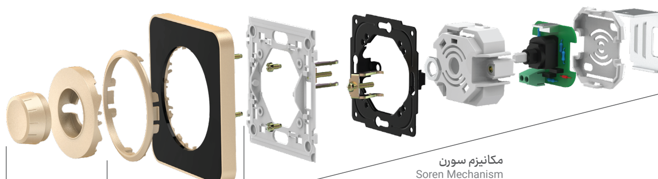
قاب رویه Decorative Frame
