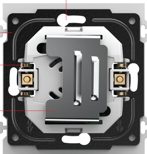
محل نصب شاسی با پیچ (بر روی دیوار کناف، MDF، و ...) Hole for mounting the chassis (on a wall of Knauf, MDF, etc.)
