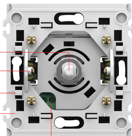
ترمینال ورودی و خروجی فاز Input and output phase terminal
