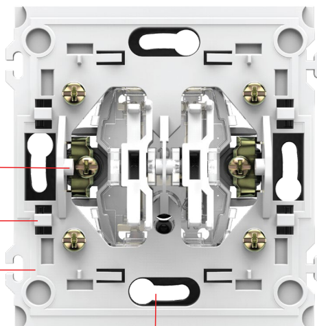
محل نصب شاسی با پیچ (بر روی دیوار کناف، MDF، ...) Hole for mounting the chassis (on a wall of Knauf, MDF, etc.)
