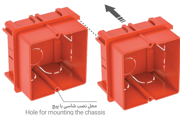
محل نصب شاسی با پیچ Hole for mounting the chassis
