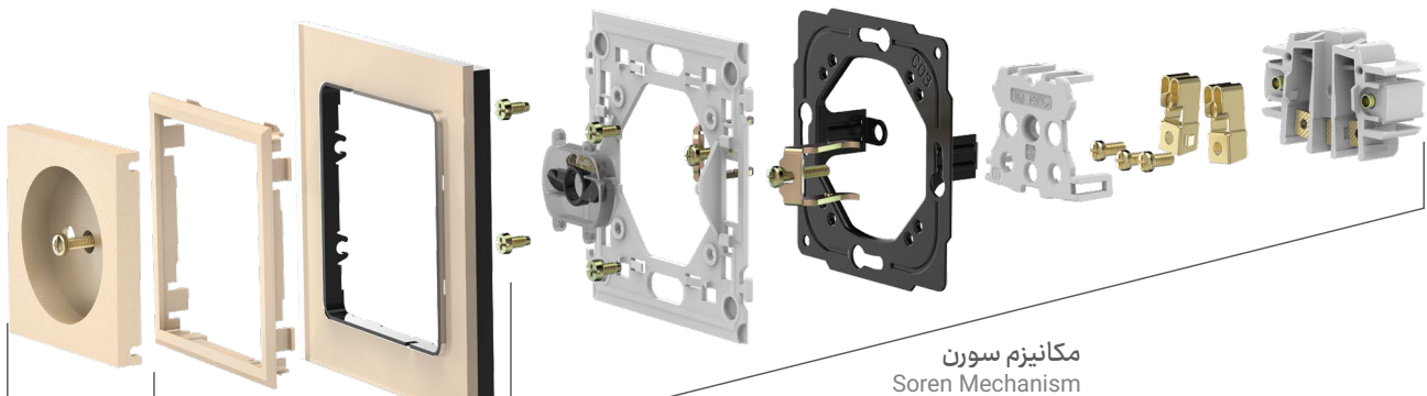
قاب رویه Decorative Frame میانی Middle cover
