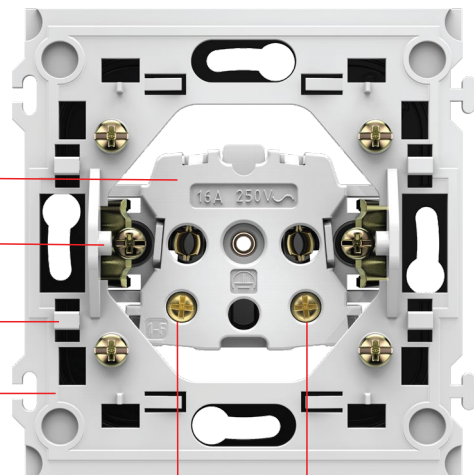
پیچ های ترمینال ورودی سیم های فاز و نول Terminal screws Input fort phase and neutral wires
